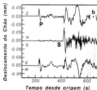
Fig. 3.3 Argentina abala São Paulo. a) Registro na estação sismográfica de Valinhos, SP, de um sismo ocorrido na fronteira Argentina/ Bolívia (23.01.1997) com magnitude 6,4. b) O movimento do chão é descrito pelos três componentes: Z (vertical, positivo para cima), NS (positivo para o Norte) e EW (positivo para o Leste). As ondas P e S chegam 230s e 410s, respectivamente, após a ocorrência do terremoto.
